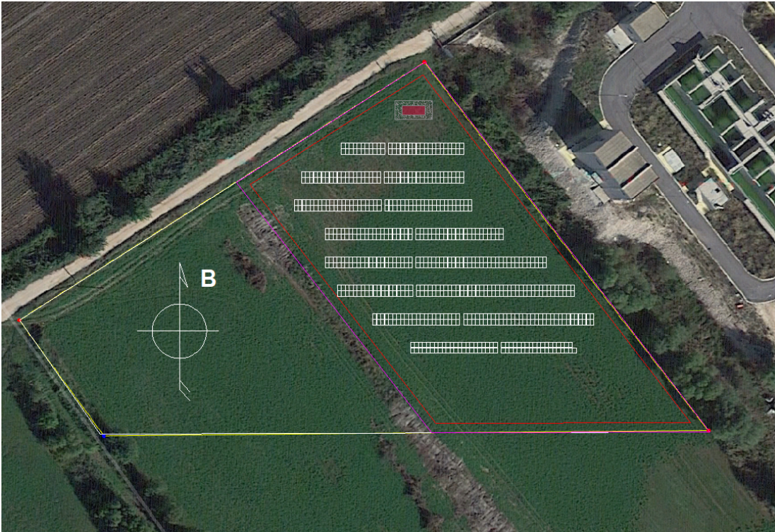
Εικόνα 3: Ενδεικτική χωροθέτηση του συστήματος επι του καθορισμένου γηπέδου. Με μωβ διακρίνονται τα όρια της περιφράξης. Με κόκκινο διακρίνεται το όριο της ζώνης εγκατάστασης βάσει των κανονισμών εγκατάστασης Φ/Β πλαισίων σε γήπεδα.
